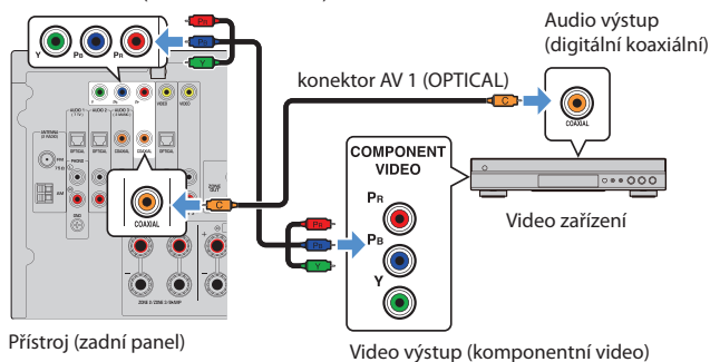
Konektor AV 1 (COMPONENT VIDEO)
